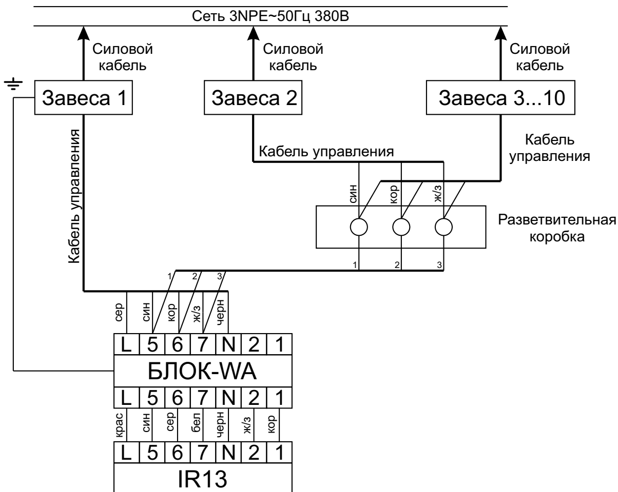
Рисунок 5.1. Схема подключения более двух завес к одному пульту управления IR13 с помощью БЛОК-WA.
