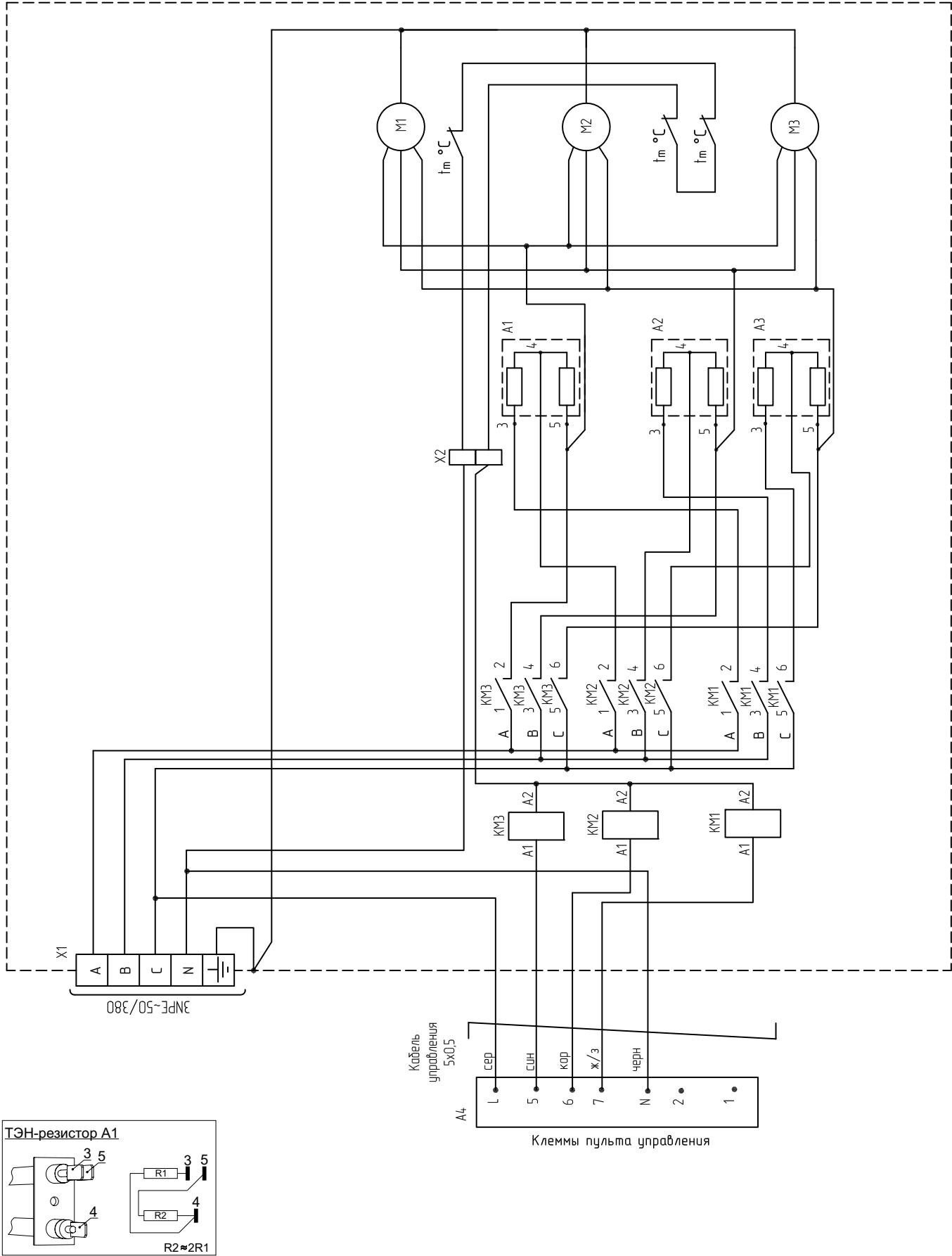
Рисунок 13. Электрическая схема занесы КЭВ-175П5060W
