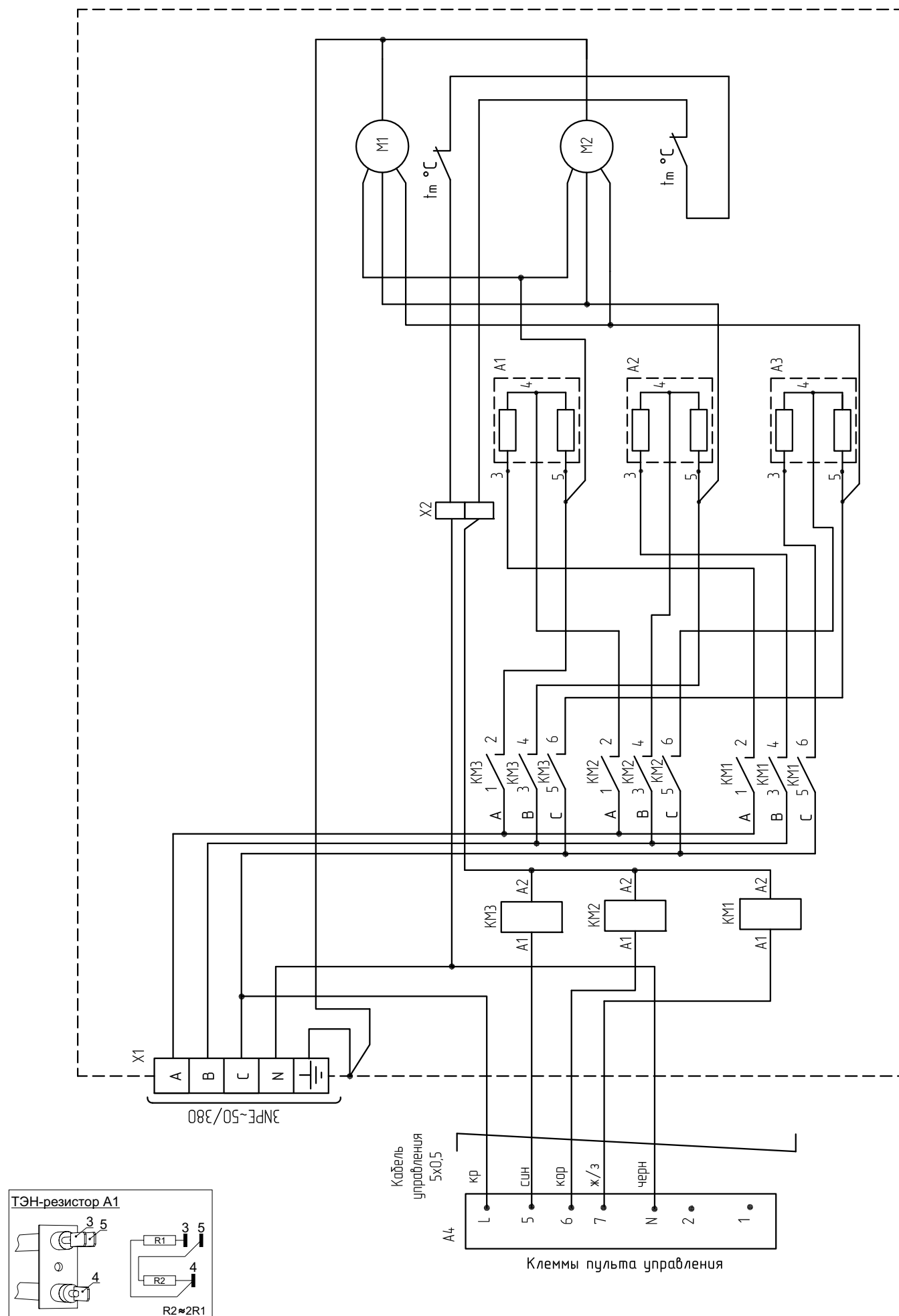
Рисунок 12. Электрическая схема занавески КЭВ-125П5050W
