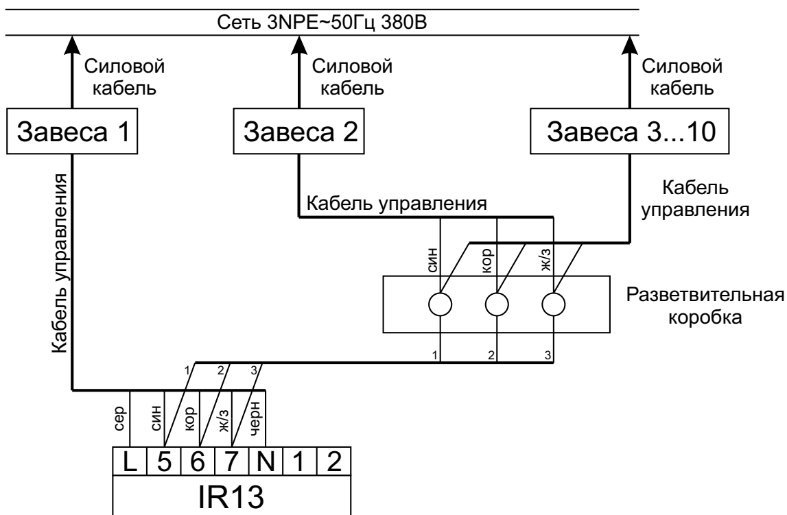
Рисунок 5.1. Схема подключения более двух завес к одному пульту управления IR13 с помощью БЛОК-WA.
