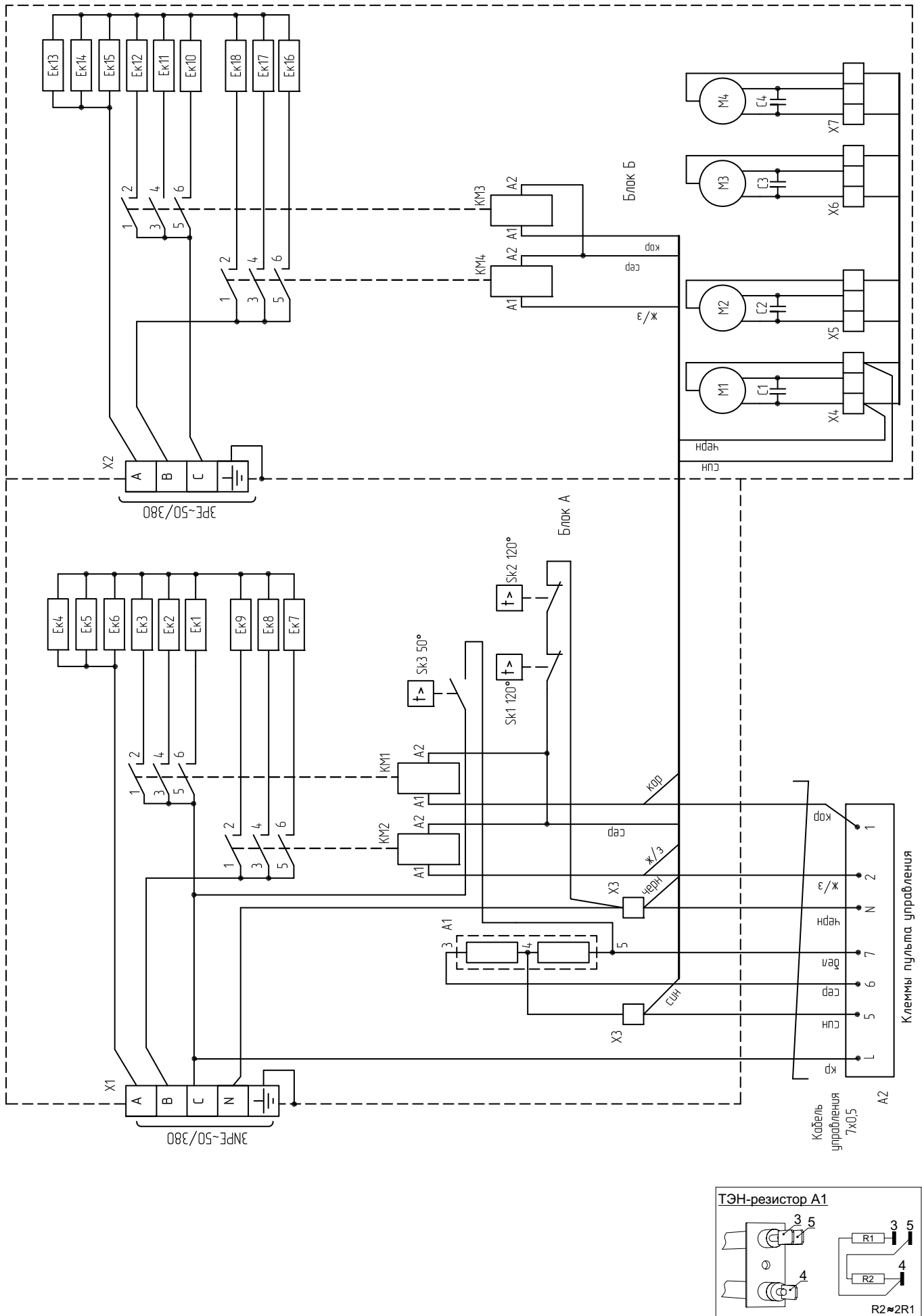
Рисунок 8. Электрическая схема завесы КЭВ-36;45П5033Е, КЭВ-54П5043Е
