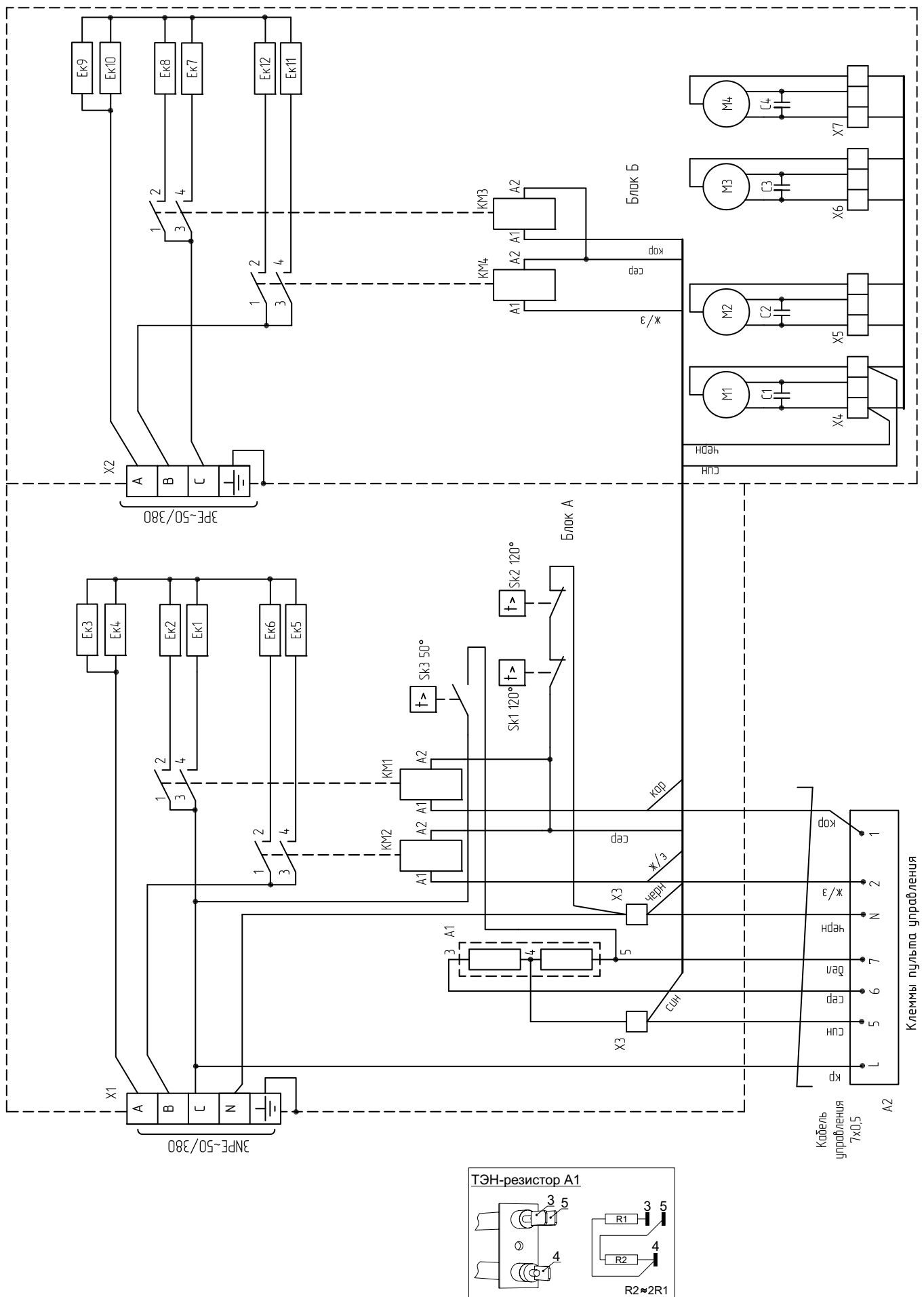
Рисунок 6. Электрическая схема завесы КЭВ-24П5033Е
