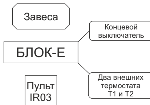
Рисунок 3. Структурная схема подключения через БЛОК-Е
