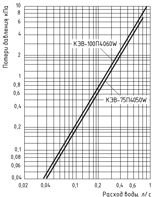
Рисунок 1. Гидравлические характеристики
